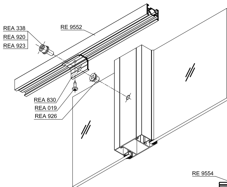
Обработка стойки
