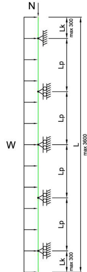
Четырехпролетная схема
