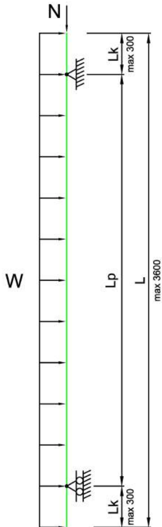
Однопролетная схема
