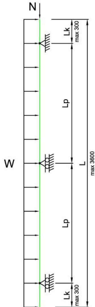
Двухпролетная схема
