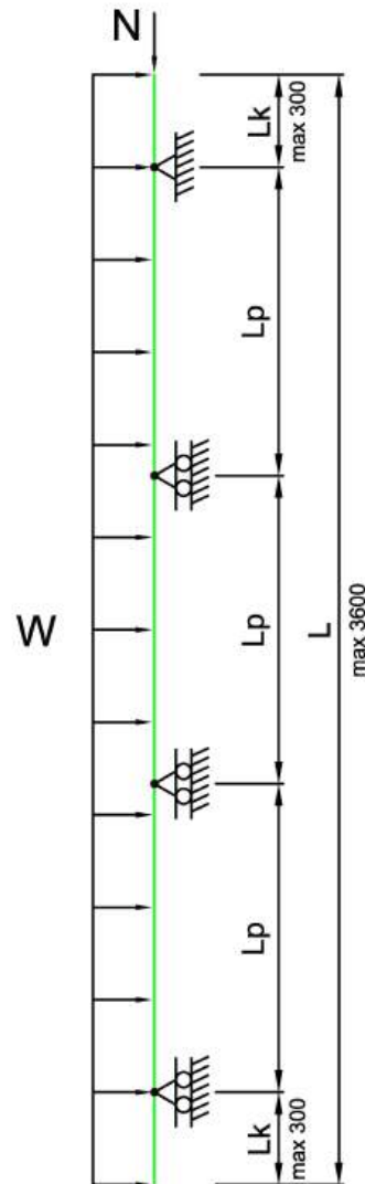
Трехпролетная схема
